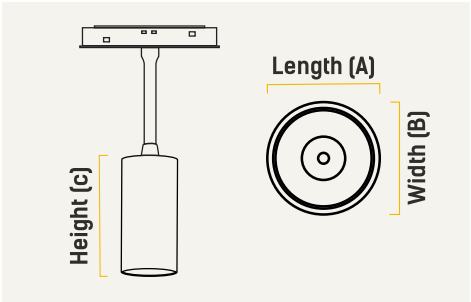
Magnetic Pendant Light
